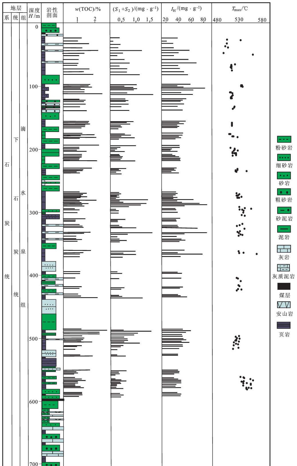
图 3 滴水泉凹陷露头 C 1d 有机地球化学剖面
