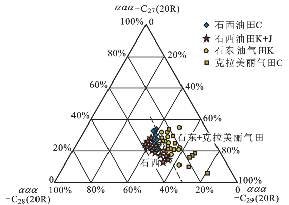
图9 石东地区原油和储层抽提物与石西、克拉美丽气田原油 C 27 -C 29 甾烷分布
