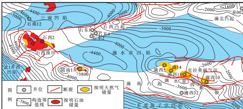
图1 滴水泉凹陷位置图
