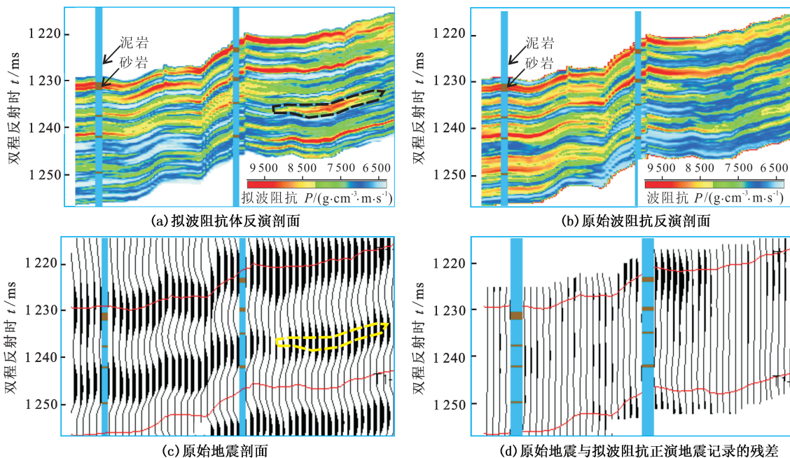
图 5 拟波阻抗体识别砂岩效果及精度分析
