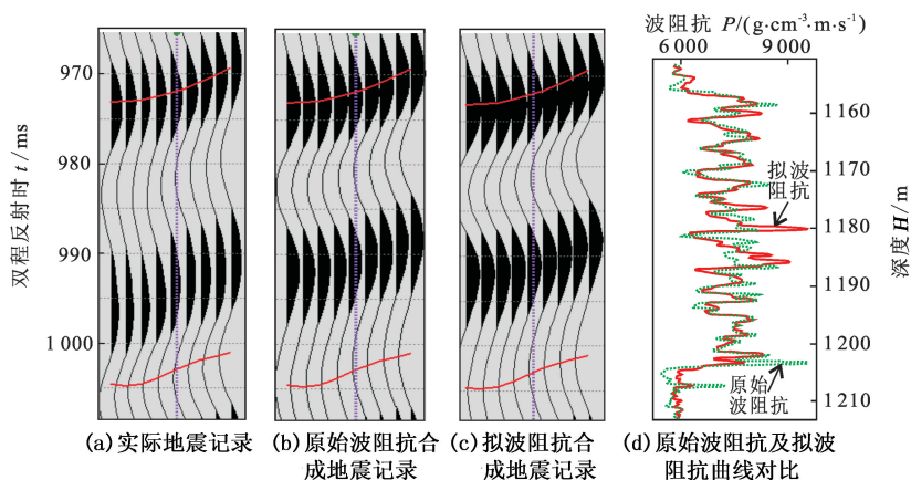
图 4 原始波阻抗、拟波阻抗曲线及合成地震记录对比
