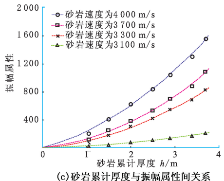
(c)砂岩累计厚度与振幅属性间关系
