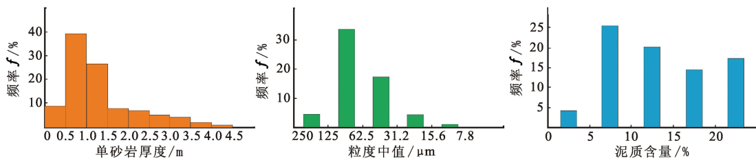
图1 敖9地区葡萄花油层单砂体厚度、粒度中值及泥质含量
