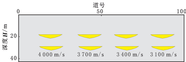
(a)不同速度的砂岩薄互层地质模型
