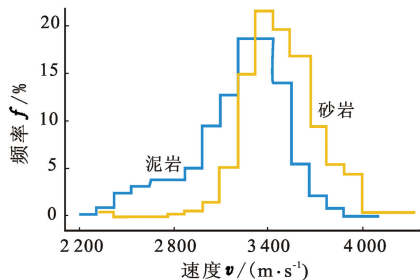
图2 敖9地区葡萄花油层砂岩和泥岩速度分布直方图
