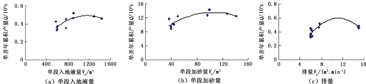
图 7 单井年累积产量与单段入地液量、加砂量、排量的关系
