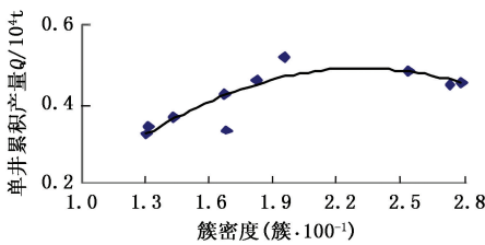
图4 压裂簇密度与单井累积产量关系
