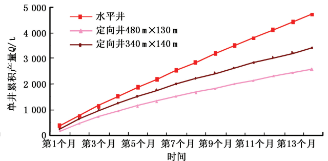
(b) 相同面积水平井与直井累积产油量
