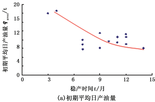
图 12 初期平均日产油量和压裂未返排液量与稳产时间关系曲线
