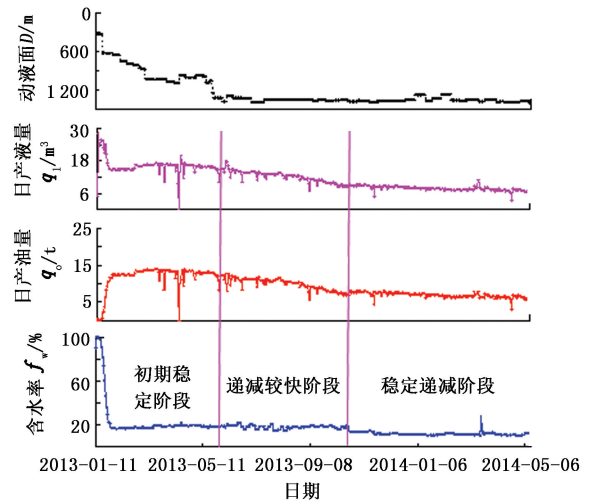
图 10 典型水平井 YP3 生产曲线
