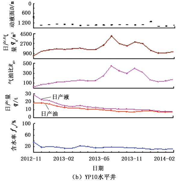
图 11 典型水平井生产动态曲线(月数据)
