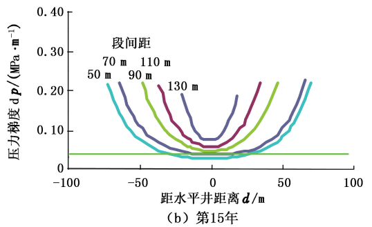
图3 不同时间地层压力梯度与段间距关系
