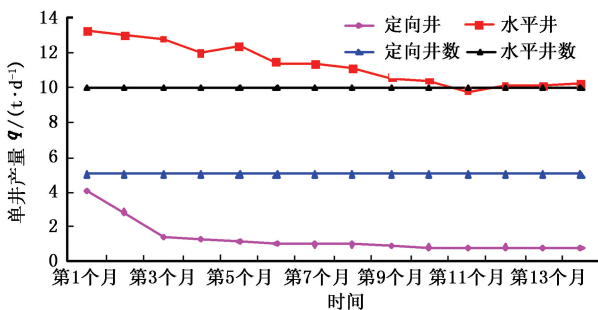
(a) 水平井与定向井单井产量
