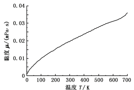
图1 氦气黏度随温度变化曲线
