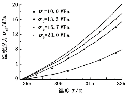
图 5 温度应力与温度的关系
