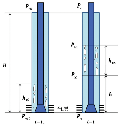
图3 关井期间气体滑脱模型示意图
