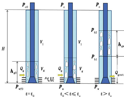
图1 关井期间井筒流体特征示意图
