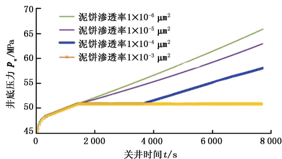
图8 泥饼渗透率对井底压力影响
