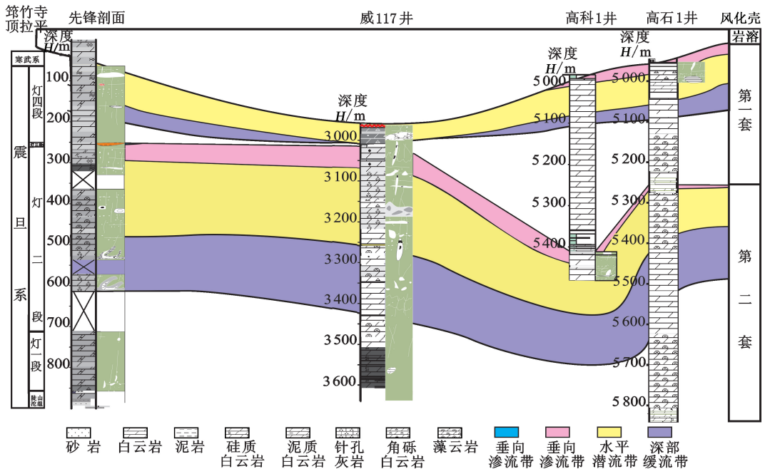
图9 四川盆地灯影组古岩溶结构横向对比
