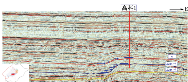
图 4 研究区高科 1 井附近上震旦系灯影组地震剖面
