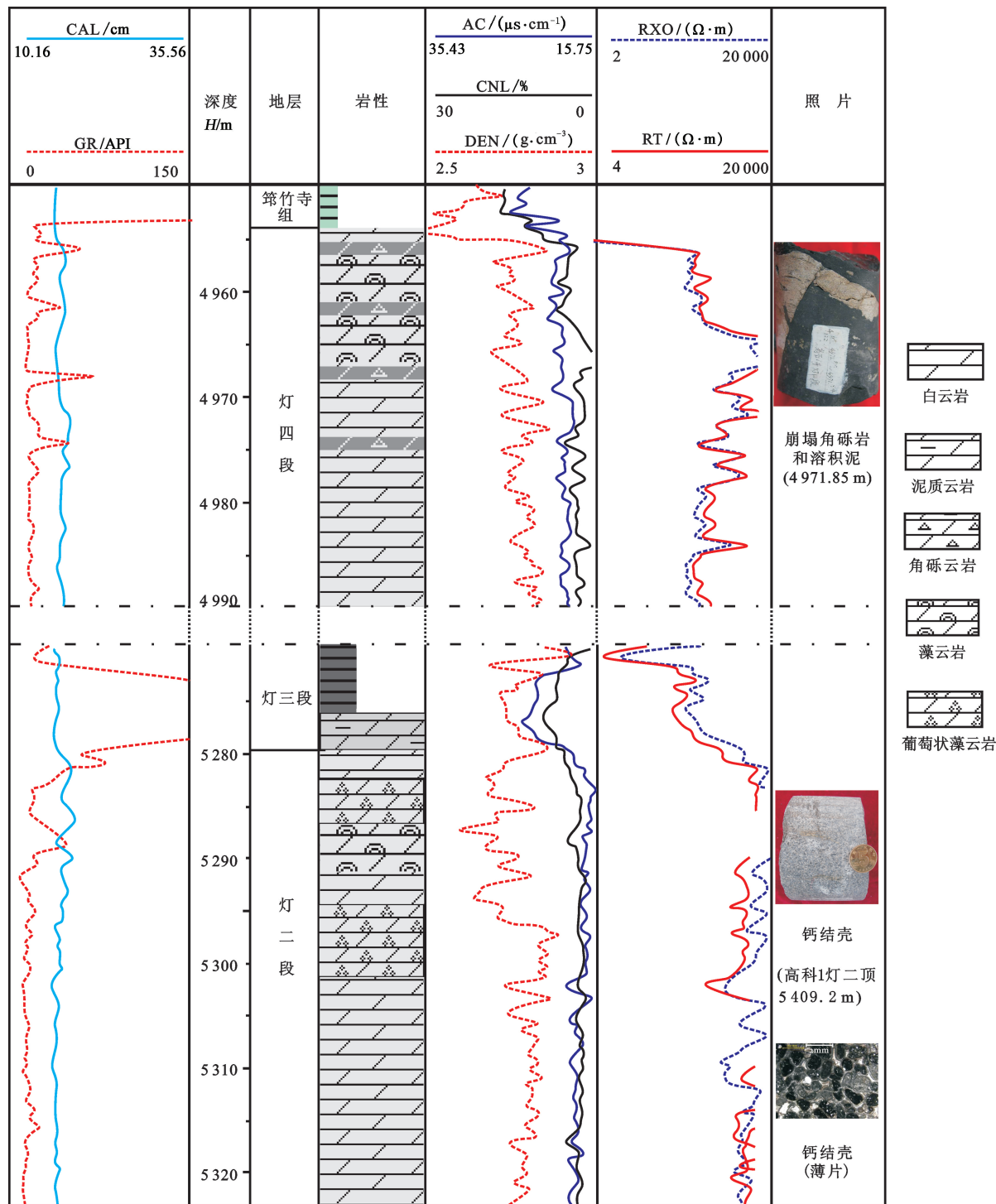
图5 高石1井灯影组测井响应与岩心特征
