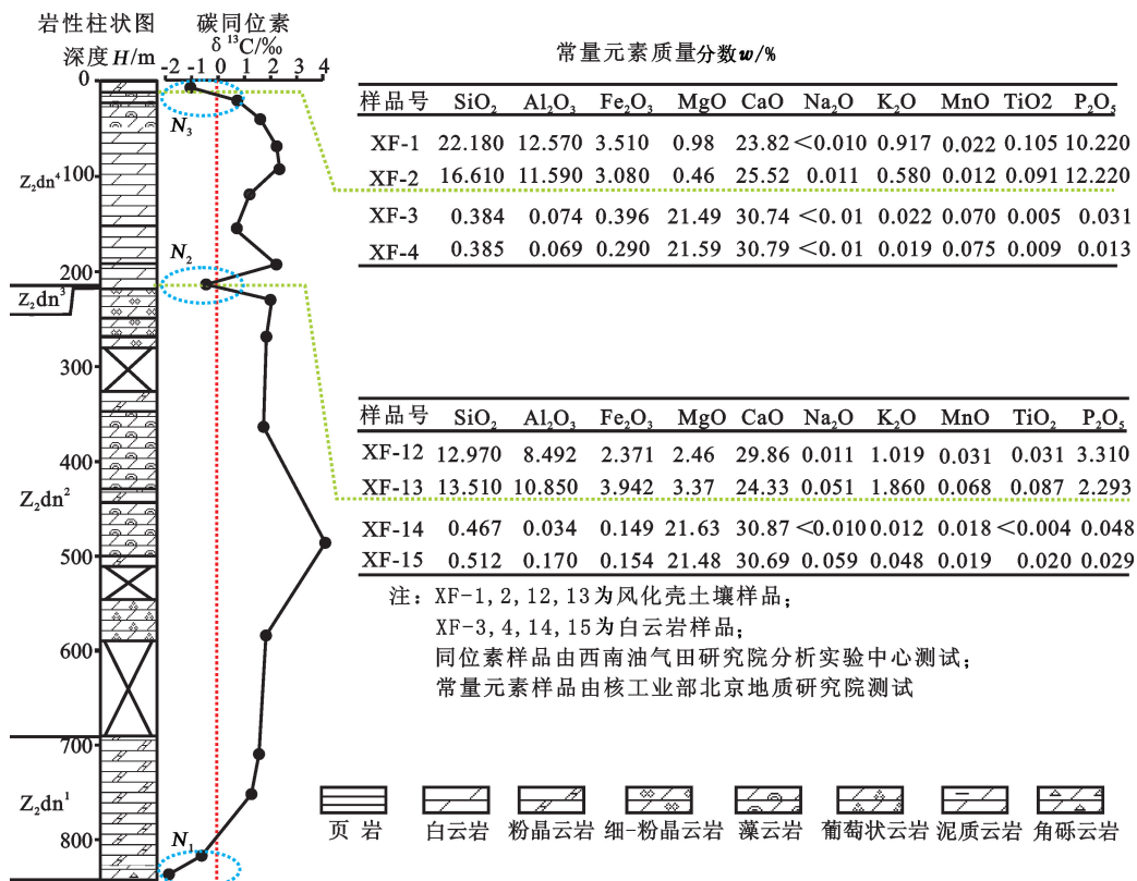
图 7 峨边先锋剖面上震旦统灯影组碳同位素及常量元素测定结果
