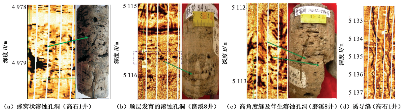
图 6 灯影组不同类型的储集空间及识别
