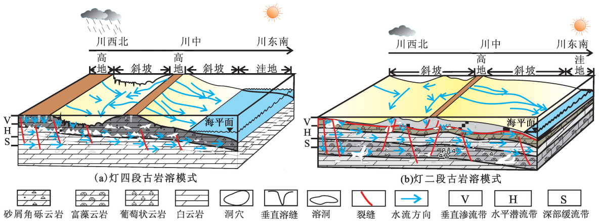
图 10 四川盆地上震旦统灯影组风化壳古岩溶模式
