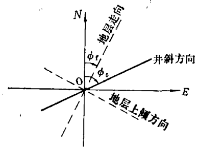
图2 水平投影图
