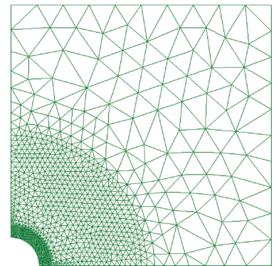
图 4 网格划分
