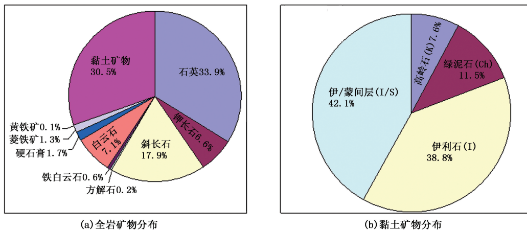
图 1 致密页岩全岩和黏土矿物分布
