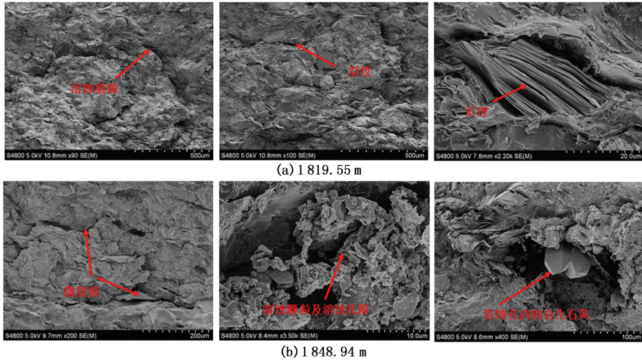
图2 岩心扫描电镜图像 Fig.2 SEM images of cores
