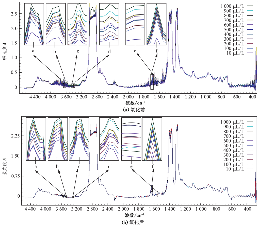
图1 热氧化实验前后不同微水含量油样的红外光谱(4700~350 cm -1 波数处)
