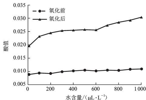
图4 热氧化实验前后不同微水含量对绝缘油酸值影响
