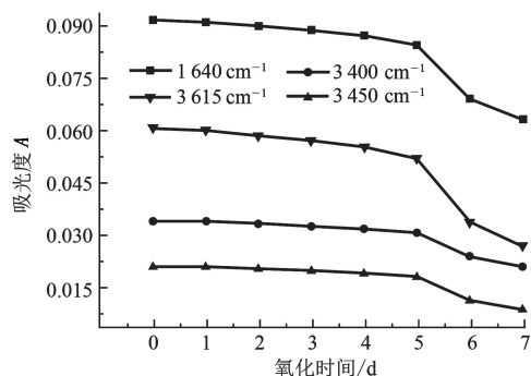
图3 10 \mu\text{L/L} 微水含量油样热氧化实验后不同波数处吸光度随热氧化时间的变化
