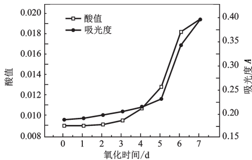
图2 10 \mu\text{L/L} 微水含量油样热氧化实验后酸值及 1700\text{ cm}^{-1} 波数处吸光度随热氧化时间的变化
