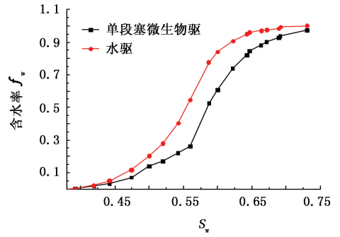
图 6 多段塞微生物含水率变化 Fig. 6 Moisture content variation of segmented slug flooding
