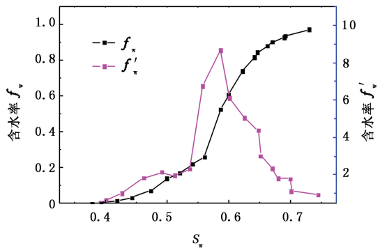
图 8 多段塞注入微生物含水率导数曲线 Fig. 8 Moisture content derivative of segmented slug flooding
