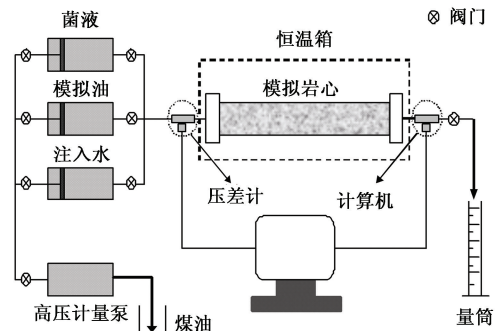
图1 岩心流动模型
