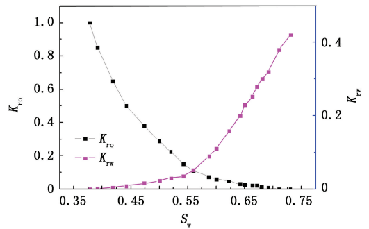
图2 现场相对渗透率曲线
