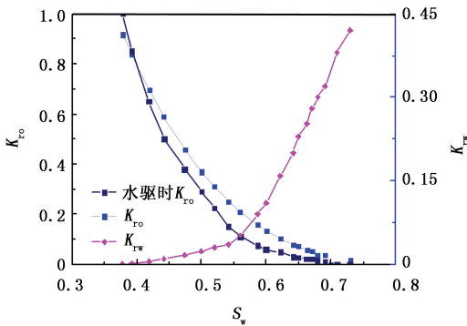
图 4 多段塞注入微生物相对渗透率曲线 Fig. 4 Relative permeability of segmented slug microbial flooding
