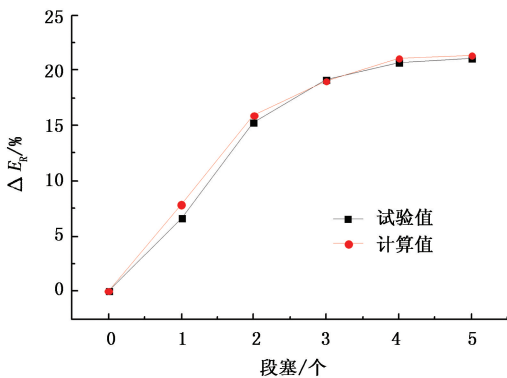
图 9 实验结果与计算结果比较
