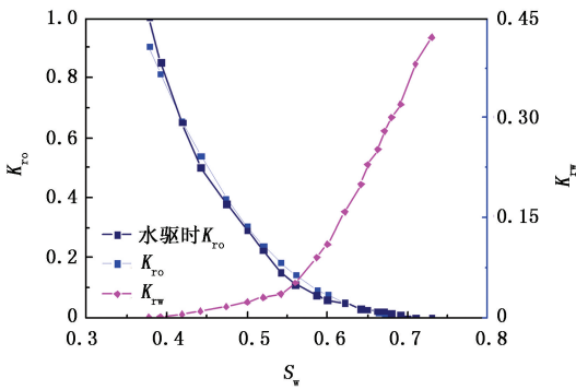
图 3 单一段塞注入微生物相对渗透率曲线 Fig. 3 Relative permeability of single slug microbial flooding
