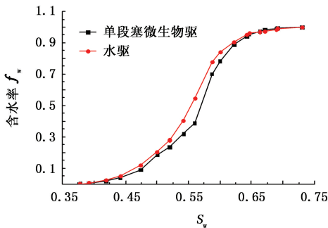
图 5 单一段塞微生物驱含水率变化 Fig. 5 Moisture content variation of single slug flooding
