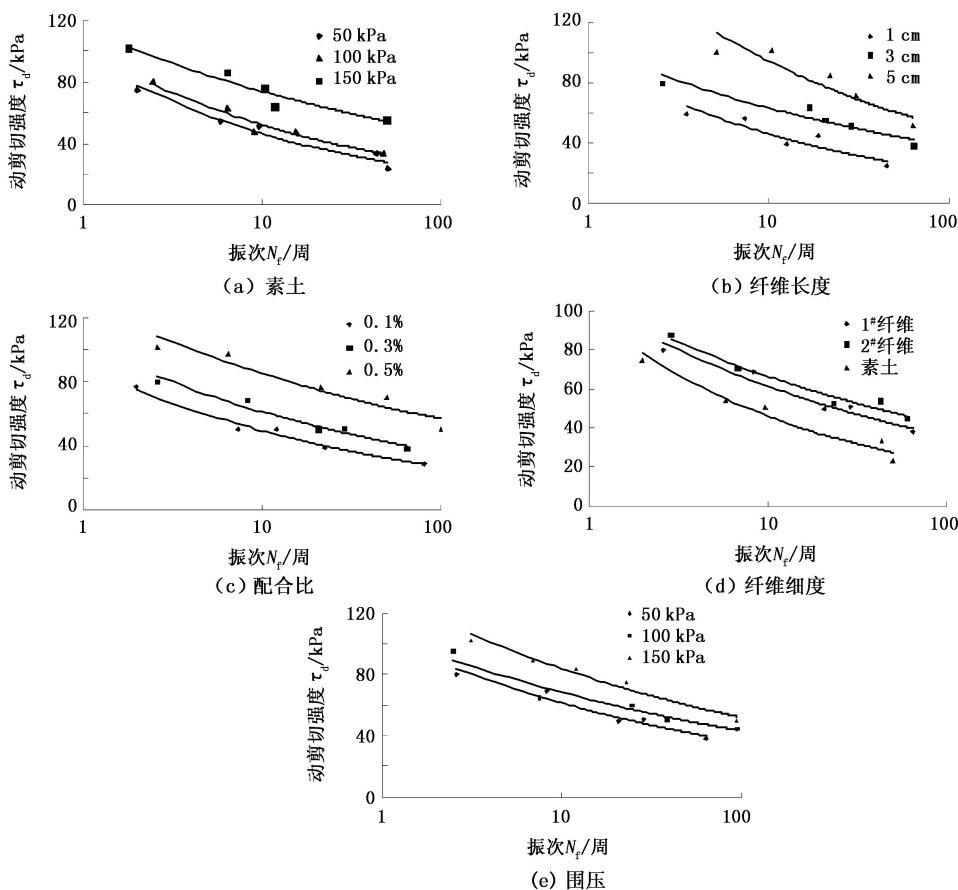
图6 纤维土 \tau_d-N_r 关系曲线
