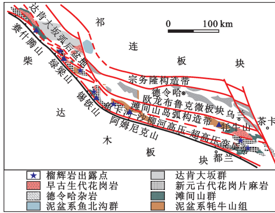
图 1 柴北缘前泥盆纪地层-构造简图
