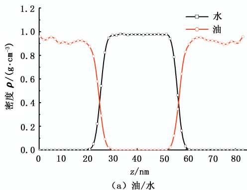
图6 油/水和NM纳米颗粒/油/水体系中各组分的密度剖面
