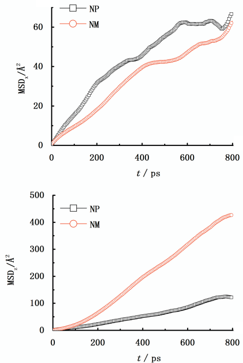
图4 纳米颗粒的均方位移
