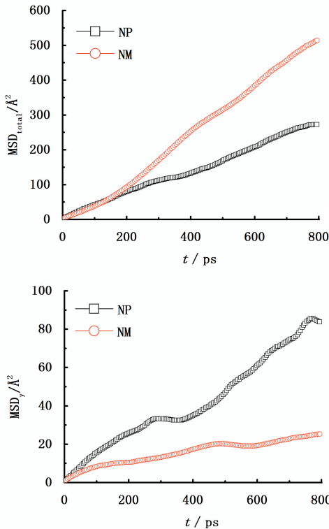
图4 纳米颗粒的均方位移
