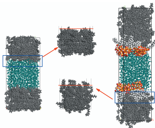
图5 体系的平衡构型
